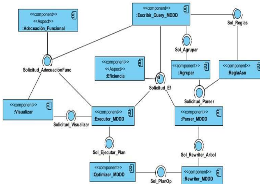
Figura 13. Arquitectura Inicial de PostgreSQLf en UML
