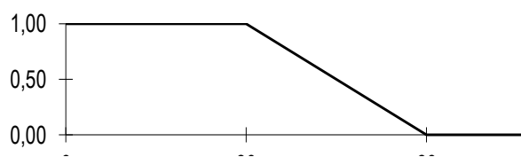
Figura 1. Definición trapezoidal del predicado difuso joven
