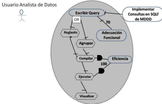
Figura 11. Modelo de Metas de PostgreSQLf en GRL
